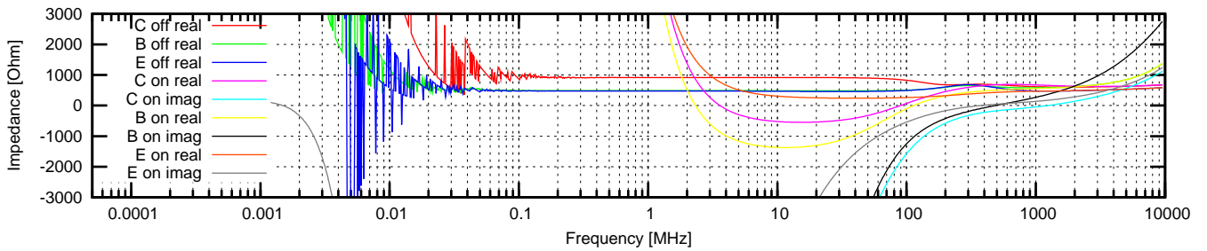
BFR 91A Worst
